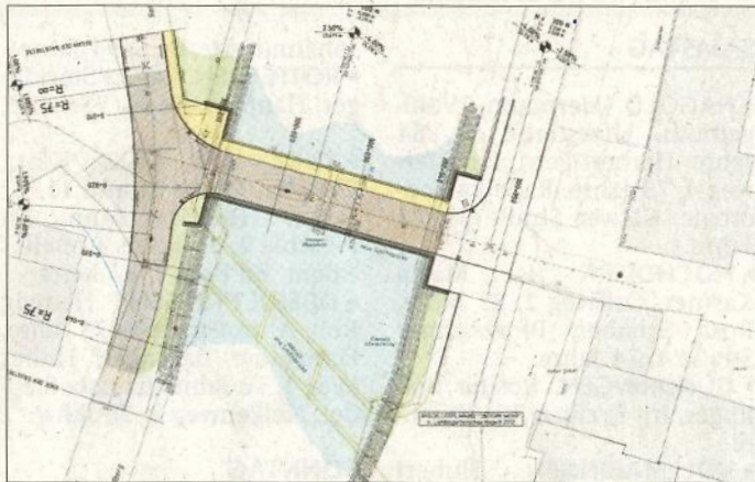
Der Plan für den Neubau der Schiffsbrücke. Die alte Brücke ist mit dünneren Linien eingezeichnet.
